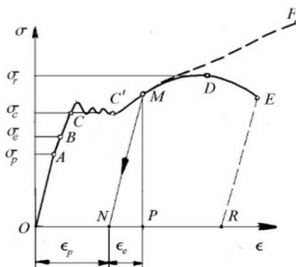
Figura 2.2. Diagrama încercării la tracțiune
